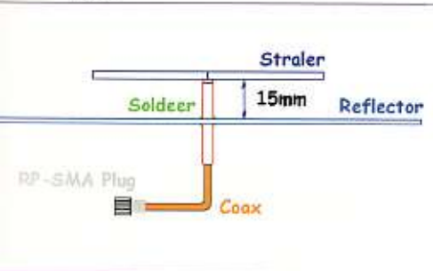
Zijaanzicht van de Biquad antenne.
